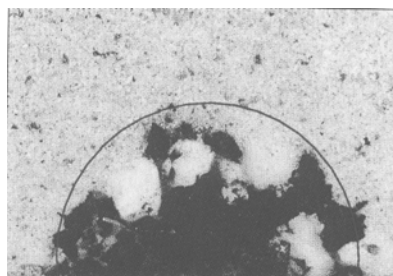
Waterstop proniká do všech trhlin a dutin. Zvětšení objemu až 300 %
